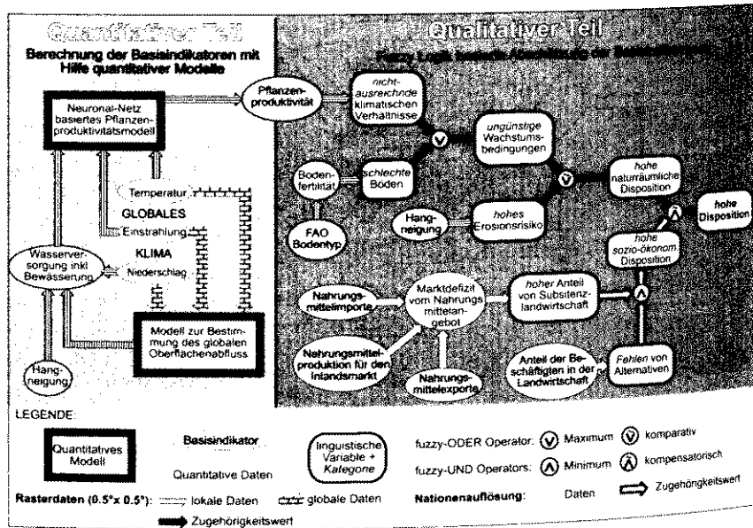
Abbildung 4: Struktur des Algorithmus zur Bestimmung der Disposition gegenüber dem Sahel-Syndrom unter Benutzung quantitativer und qualitativer Modellelemente.
