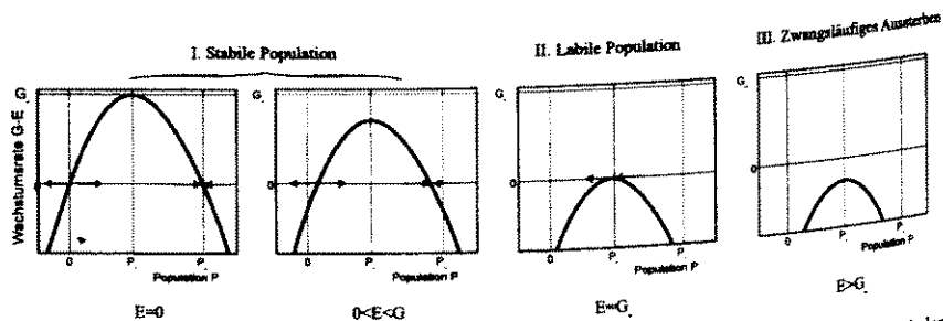
Abbildung 6: Darstellung der verschiedenen Fälle für das Verhältnis des Wachstums und der Entnahme aus dem System in der quantitativen Form unseres didaktischen Modells. Dargestellt sind jeweils das Wachstum als Funktion der Population und die jeweiligen Fixpunkte, wobei die Pfeile die Art des Fixpunktes (stabil/labil) charakterisieren.
