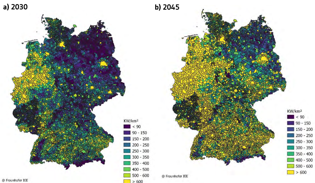
Abbildung 5.12: Installierte Leistung in kW/km 2 von PV-Aufdachanlagen für jede Gemeinde in Deutschland für das Fokus PV-Szenario.
