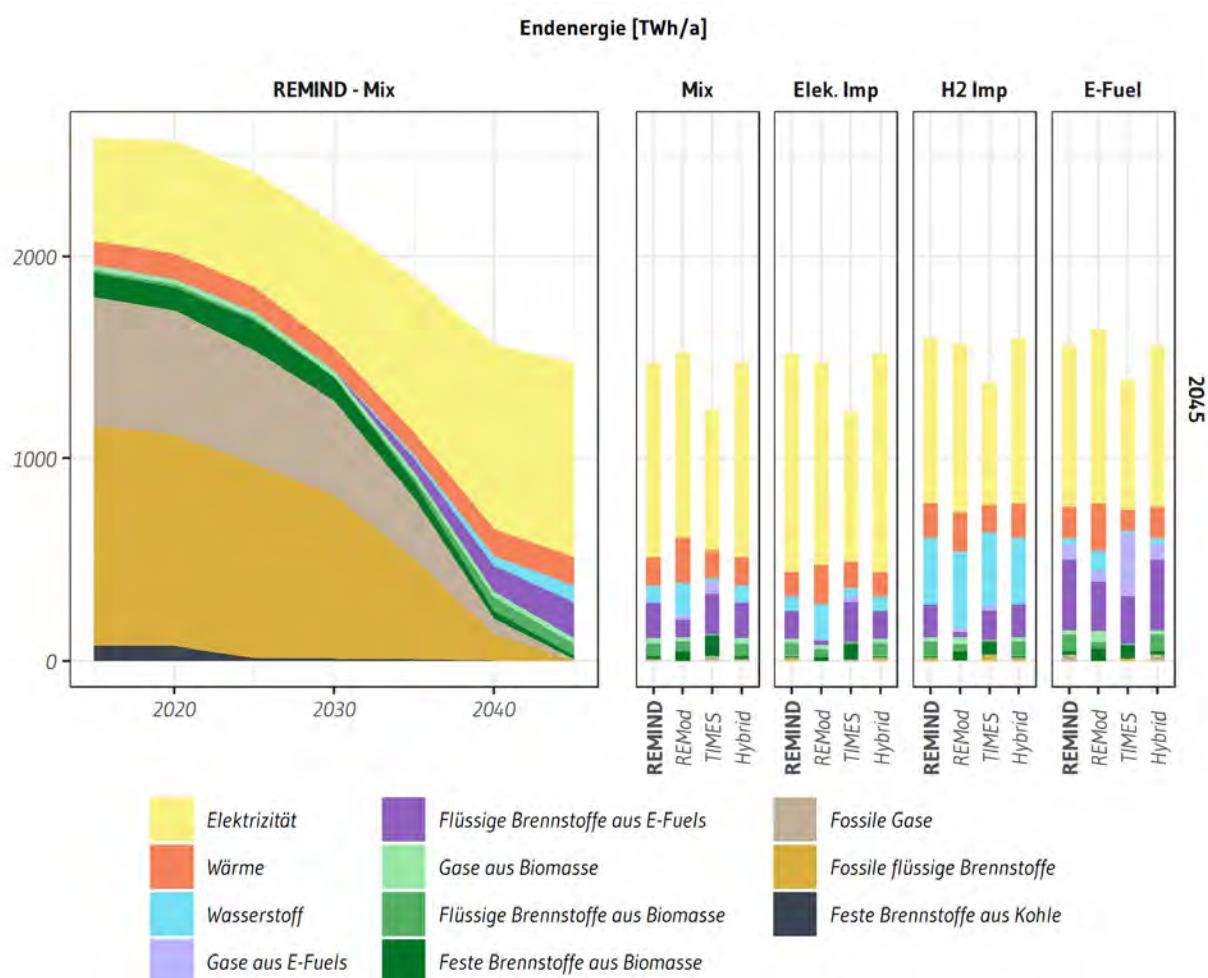
Abbildung 1.8: Endenergienachfrage inklusive stofflicher Nutzung aufgeschlüsselt nach Sektoren und Energieträgern in den verschiedenen Szenarien. Links: REMIND-Ergebnisse für den Zeitraum 2015 bis 2045 im Technologiemix-Szenario. Rechts: Ergebnisse der Gesamtsystemmodelle und dem Hybrid-Modell für verschiedene Technologieszenarien in 2030 und 2045.
