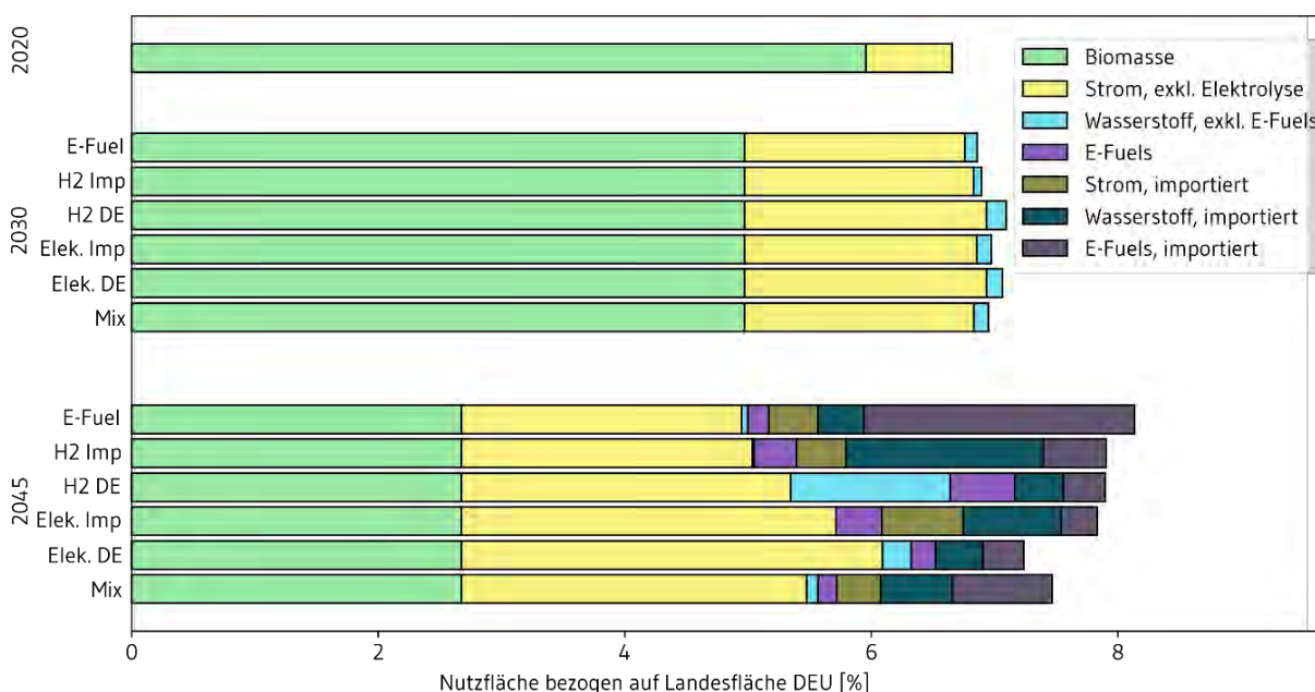
Abbildung 9.9: Gesamter Flächenbedarf weltweit von Anbaubiomasse, Strom (aus Wind und PV), Wasserstoff (aus Elektrolyse) und synthetischen Kraftstoffen bezogen auf die Landesfläche Deutschlands für die Jahre 2020, 2030 und 2045 und für alle betrachteten Szenarien.
