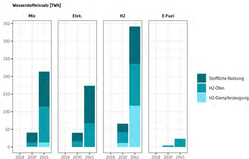
Abbildung 4.8: Wasserstoffesinsatz nach Szenario und Anwendung (2018 – 2045, TWh). Quelle: Fraunhofer ISI - FORECAST Modell.
