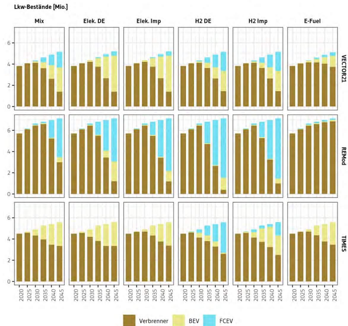
Abbildung 2.5: Lkw-Bestandsentwicklungen für die Technologiepfade bis 2045.
