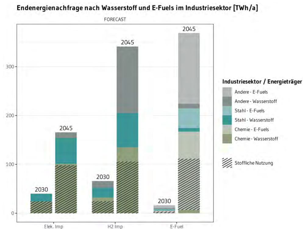
Abbildung 6.6: Nachfragen nach Wasserstoff und E-Fuels des Industriesektors in 2030 und 2045.
