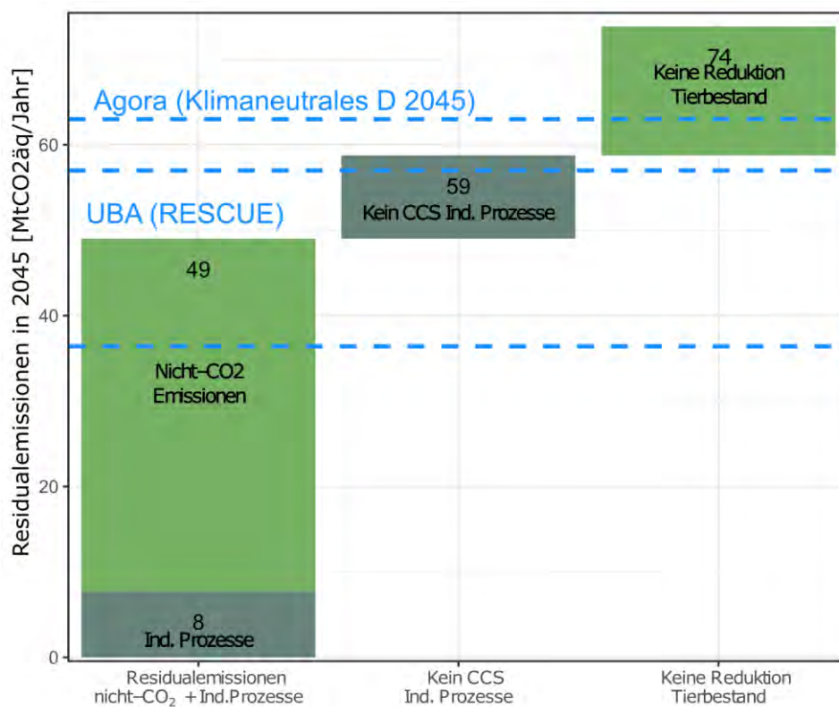
Abbildung 8.1: Residualemissionen in 2045 im Szenario TechnologiemiX unter verschiedenen Annahmen. Falls CCS für Emissionen aus Industrieprozessen zur Verfügung steht und die Tierbestände stark reduziert werden, können die Restemissionen auf ca. 49 MtCO 2 äq/Jahr gesenkt werden. Ohne CCS und mit einer geringeren Reduktion der Tierbestände kommen 10 bzw. 15 MtCO 2 äq/Jahr dazu, so dass die Restemissionen dann bei 74 MtCO 2 äq/Jahr lägen. CCS-Emissionen basieren auf Berechnungen mit dem Modell FORECAST, nicht-CO 2 -Emissionen auf dem Modell REMIND. Im Vergleich werden die Residualemissionen aus der Studie „Klimaneutrales Deutschland 2045“ (Prognos, Öko-Institut, Wuppertal-Institut et al., 2021) und die Bandbreite aus der RESCUE-Studie des UBA (UBA, 2019) gezeigt.
