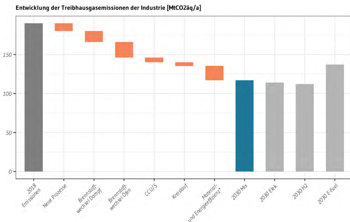
Abbildung 4.9: Beitrag einzelner Vermeidungsoptionen zur Emissionsminderung bis zum Jahr 2030 gegenüber 2018 im Szenario Technologiemit. Quelle: Fraunhofer ISI – FORECAST Modell.
