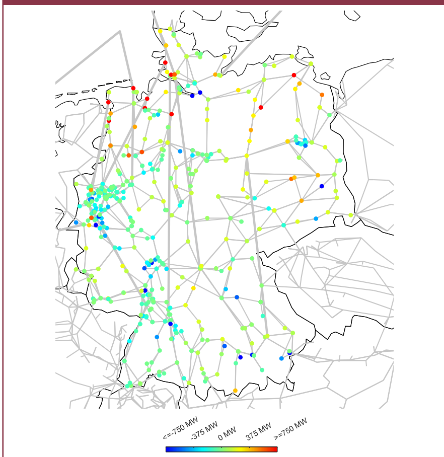
Abbildung 19: Regionale Belastungen von Verbrauch und Erzeugung im Jahr 2045 (Netto-Export) je Netzknoten. Quelle: Eigene Darstellung
