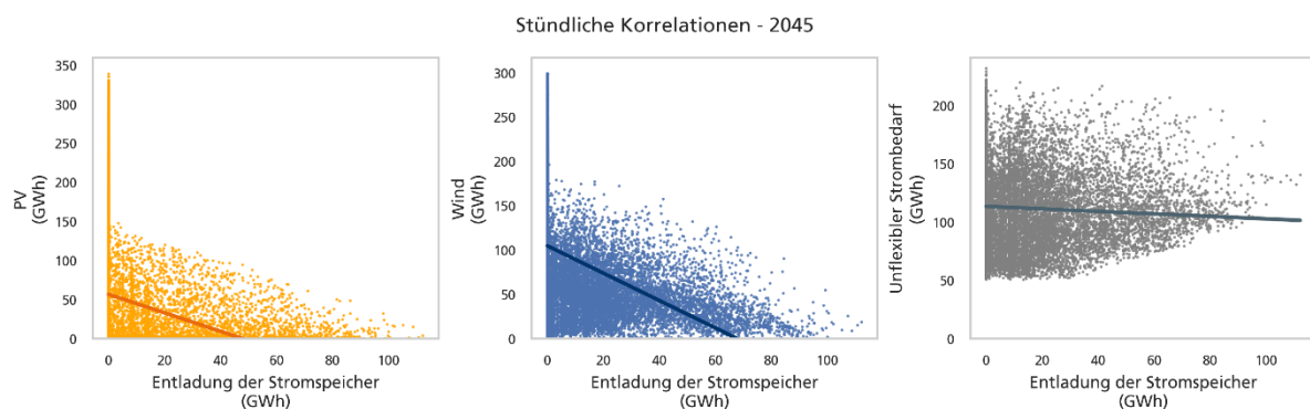
Abbildung 17: Korrelationen der Speicherentladung im Jahr 2045
