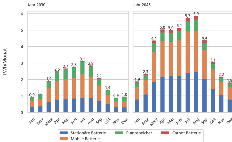
Abbildung 13: Monatsauswertung der Entlademengen von Energiespeichern in den Jahren 2030 und 2045
