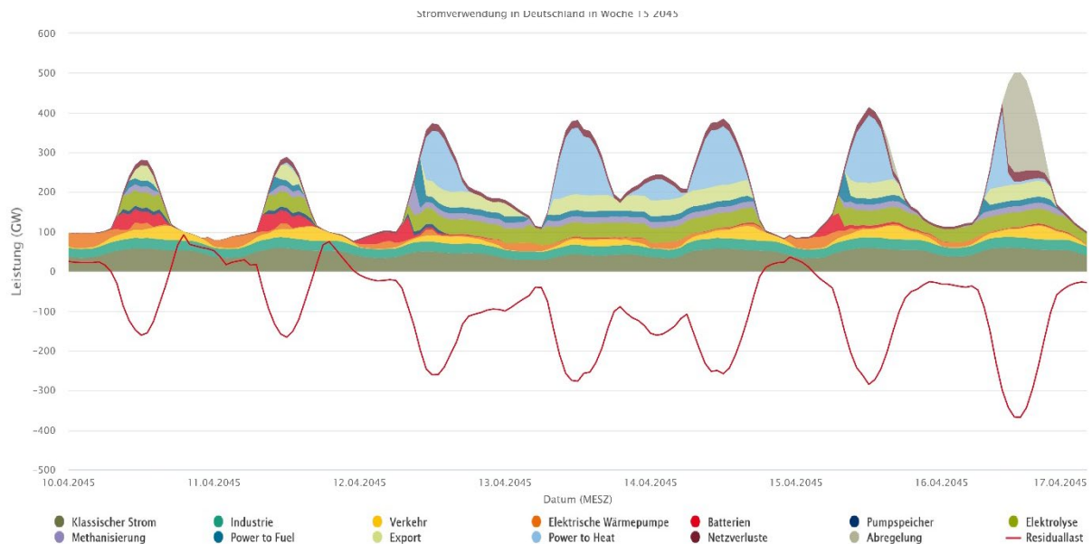
Abbildung 7: Beispielhafte Darstellung der Stromverwendung in Deutschland in der Kalenderwoche 15 im Jahr 2045
