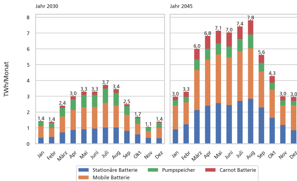
Abbildung 12: Monatsauswertung der Einspeicherungsmenge an Strom in Energiespeichern in den Jahren 2030 und 2045
