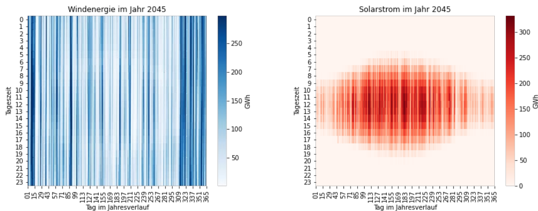
Abbildung 3: Windenergie- und Solarstromerzeugung im Jahr 2045
