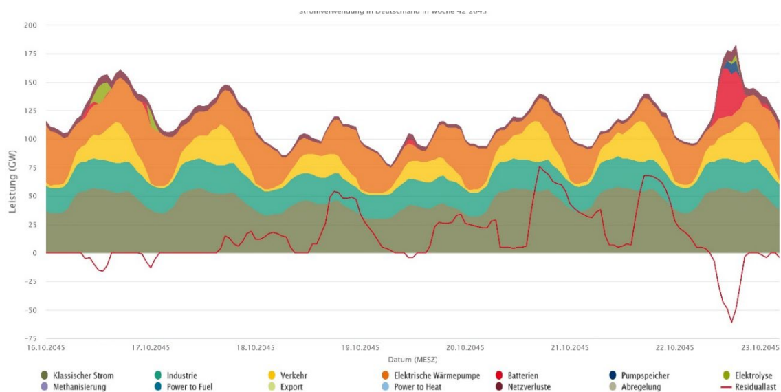
Abbildung 9: Beispielhafte Darstellung der Stromverwendung in Deutschland in der Kalenderwoche 42 im Jahr 2045
