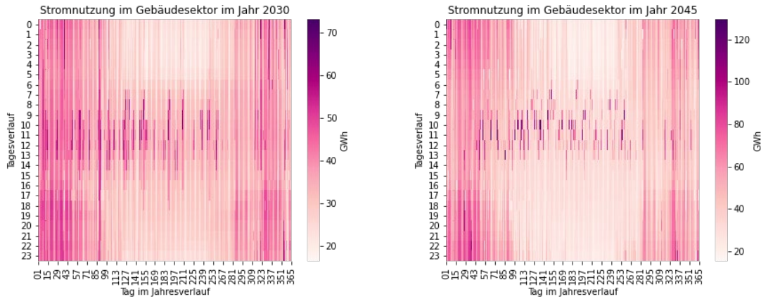
Abbildung 25: Stromnutzung im Gebäudesektor in den Jahren 2030 und 2045
