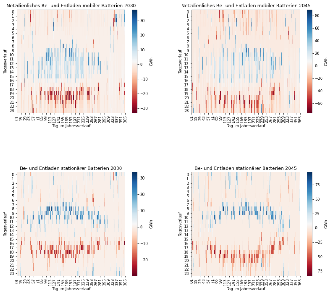
Abbildung 14: Betriebsstunden für netzdienliche Be- und Entladung von stationären (unten) und mobilen (oben) Batterien im zeitlichen Verlauf für 2030 und 2045 (positive Werte stehen für Ladevorgänge, negative Werte für Entladevorgänge)
