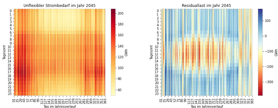
Abbildung 4: Zu deckender Strombedarf und Residuallast im Jahr 2045
