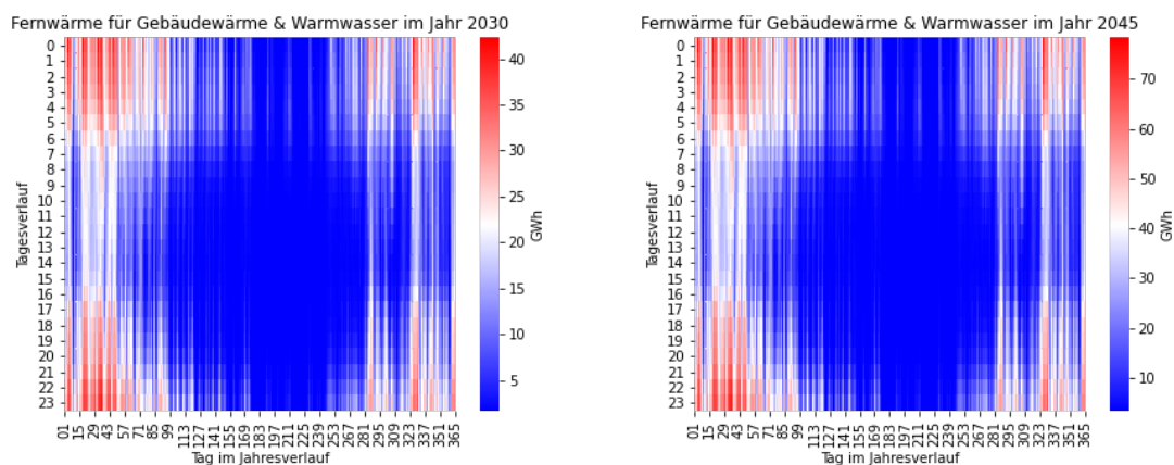
Abbildung 26: Nutzbare Fernwärme für Gebäudewärme und Warmwasser in den Jahren 2030 und 2045
