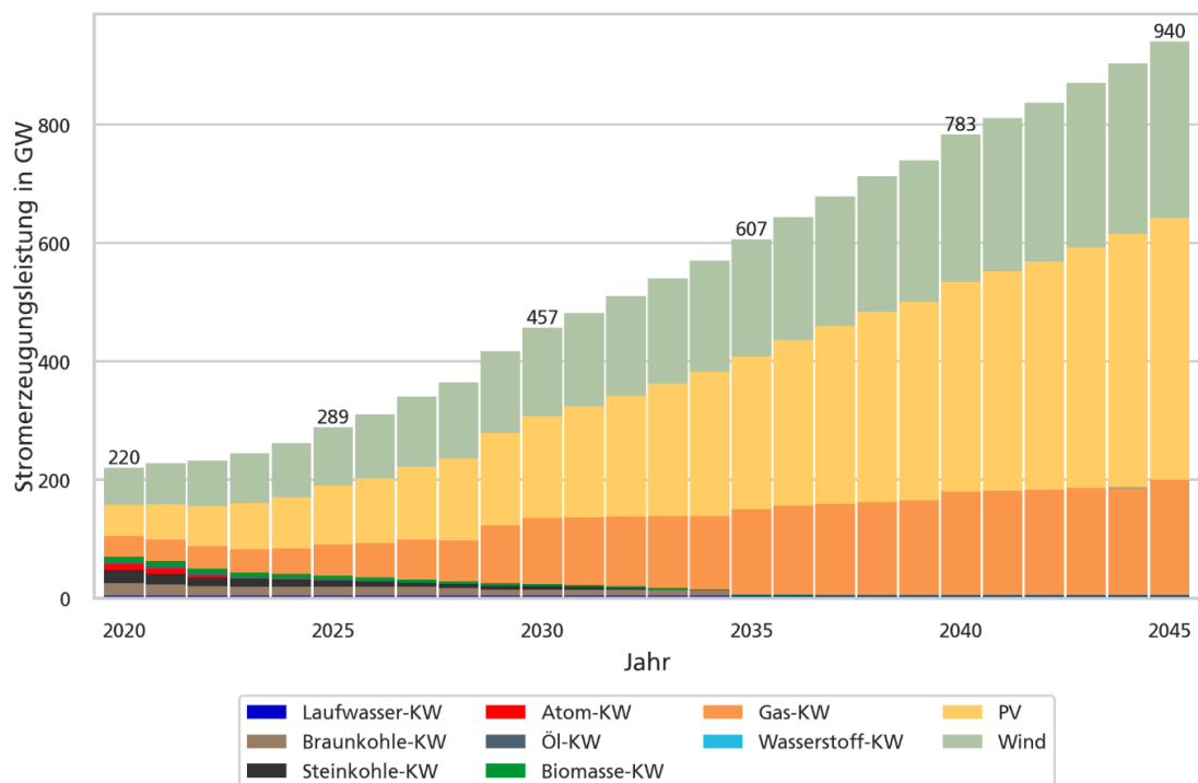
Abbildung 1: Entwicklung der Stromerzeugungsleistung im Balanced-Szenario von 2020 bis 2045 in GW (berechnet mit REMod)
