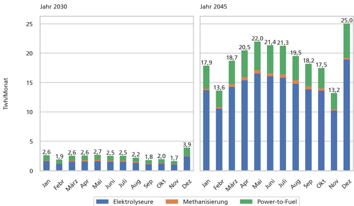
Abbildung 20: Flexibilitätsbeiträge der Power-to-X-Technologien zur Herstellung von Wasserstoff (Elektrolyseure), SynGas (Methanisierung) und eFuels (Power-to-Fuel) in den Jahren 2030 und 2045.
