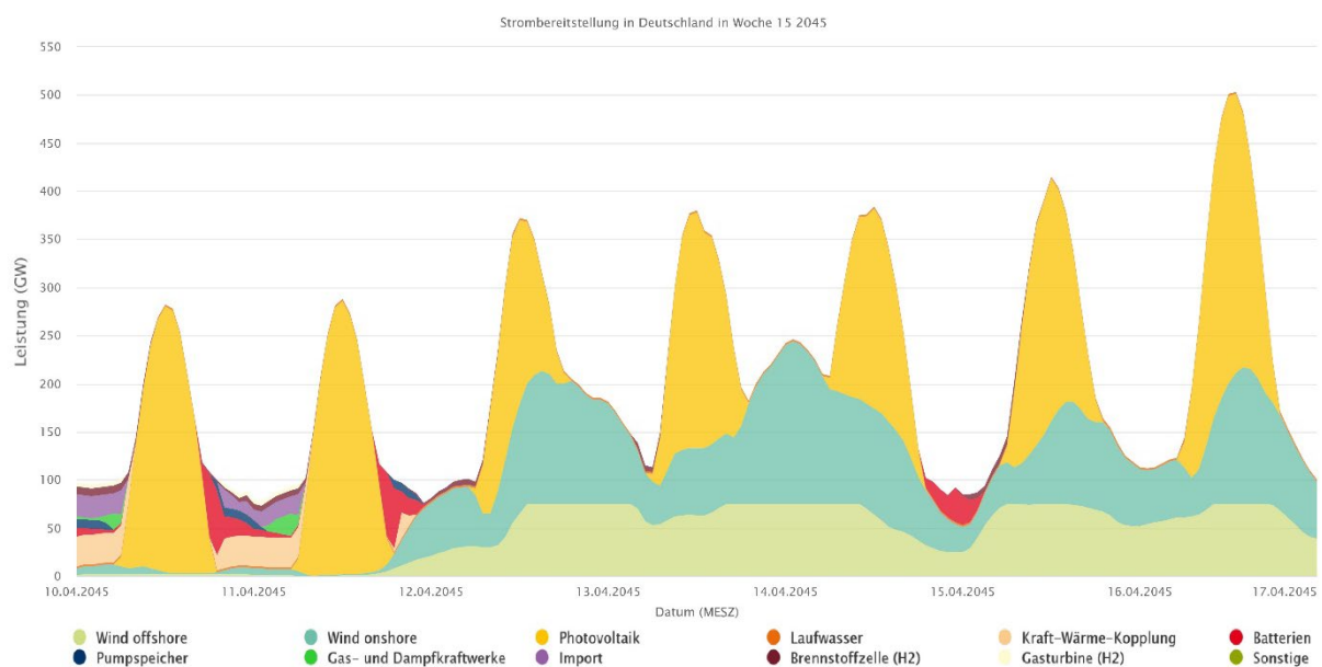
Abbildung 6: Beispielhafte Darstellung der Strombereitstellung in Deutschland in der Kalenderwoche 15 im Jahr 2045
