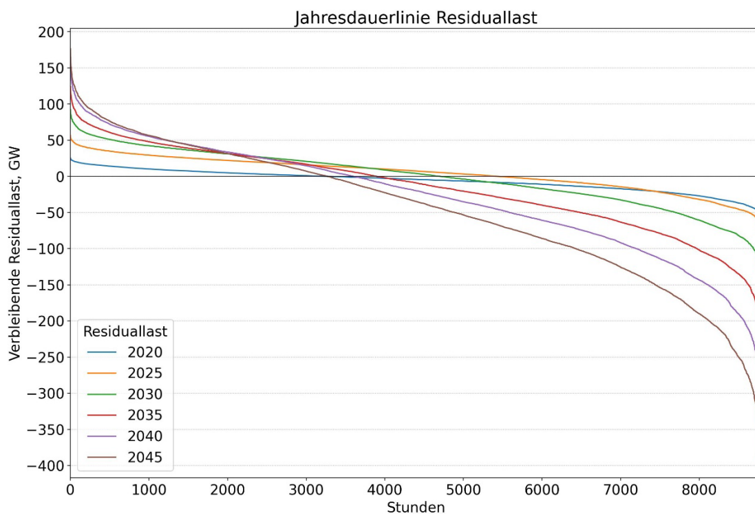
Abbildung 5: Jahresdauerlinien der Residuallast
