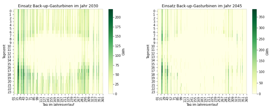
Abbildung 29: Betrieb von Backup-Gasturbinen im Jahresverlauf in den Jahren 2030 und 2045
