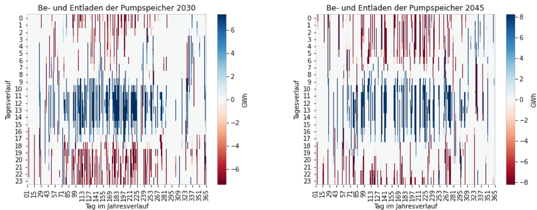
Abbildung 15: Betriebsstunden für Be- und Entladung für Pumpspeicherkraftwerke im zeitlichen Verlauf für 2030 und 2045
