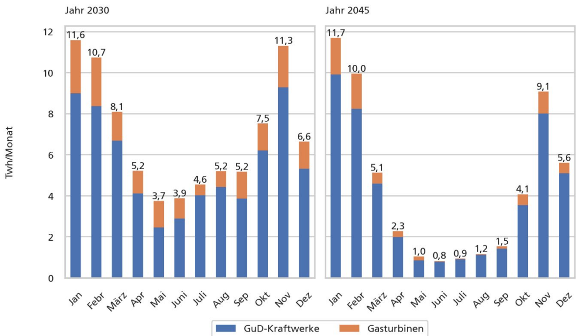
Abbildung 28: Beitrag flexibler Gaskraftwerke (GuD und Gasturbinen) zum Lastausgleich in den Jahren 2030 und 2045. Gaskraftwerke können dabei sowohl mit Erdgas als auch mit biogenem oder synthetischem Gas sowie Wasserstoff betrieben werden.
