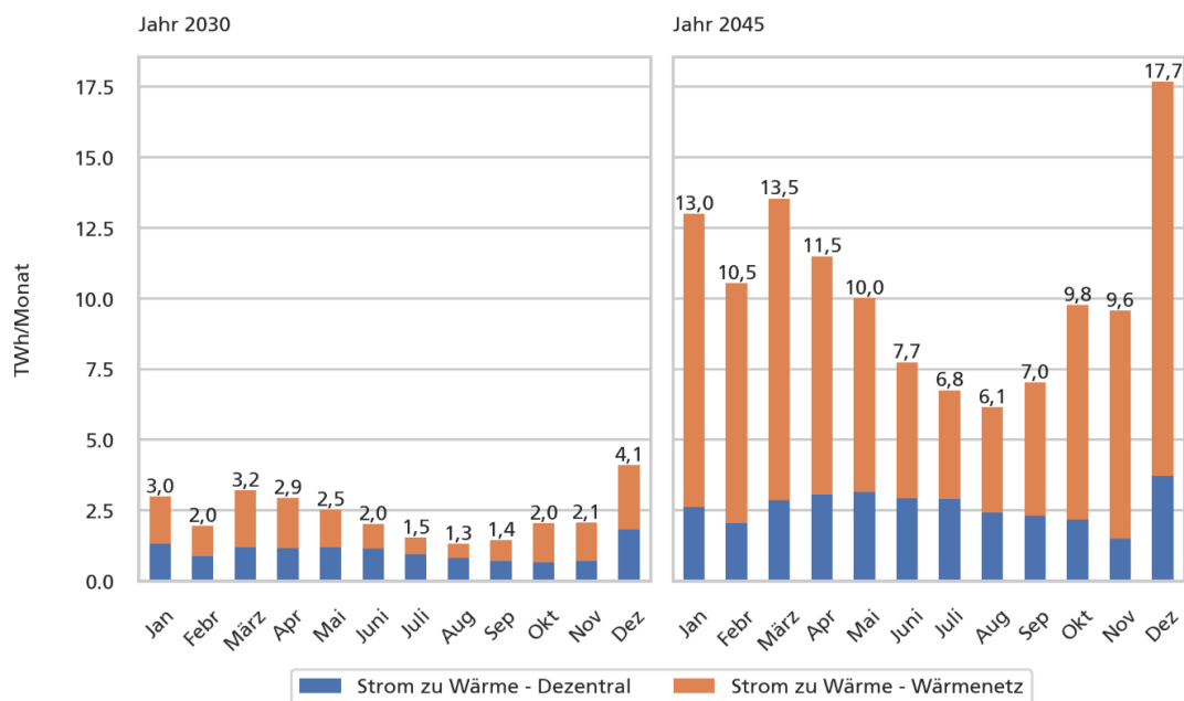
Abbildung 24: Dezentrale und zentrale Wärmeversorgung durch Strom in den Jahren 2030 und 2045.
