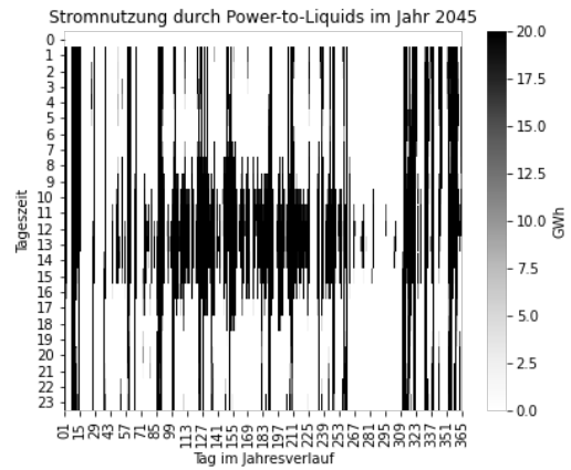
Abbildung 22: Stromverwendung durch Power-to-Fuel im Jahr 2045
