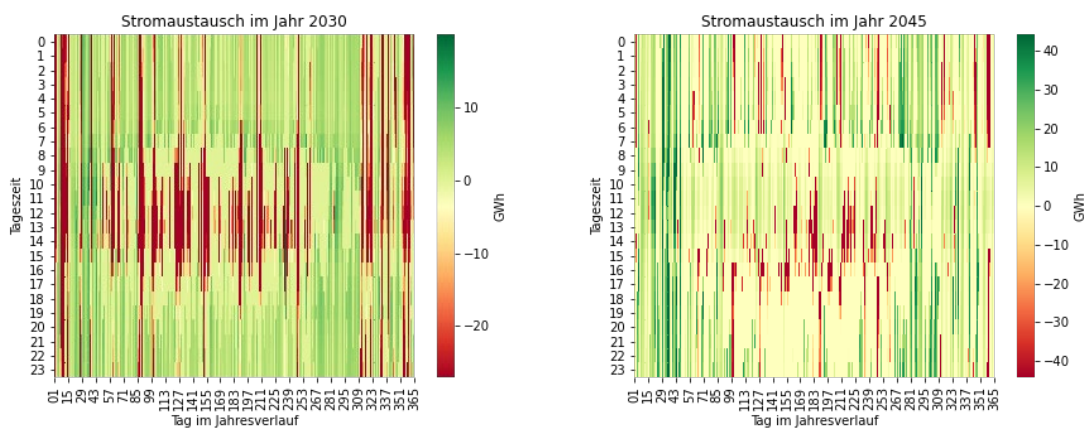
Abbildung 27: Stromimporte und -exporte in den Jahren 2030 und 2045. Positive Werte stellen Stromimport nach Deutschland, negative Werte Stromexport aus Deutschland in die Nachbarländer dar.
