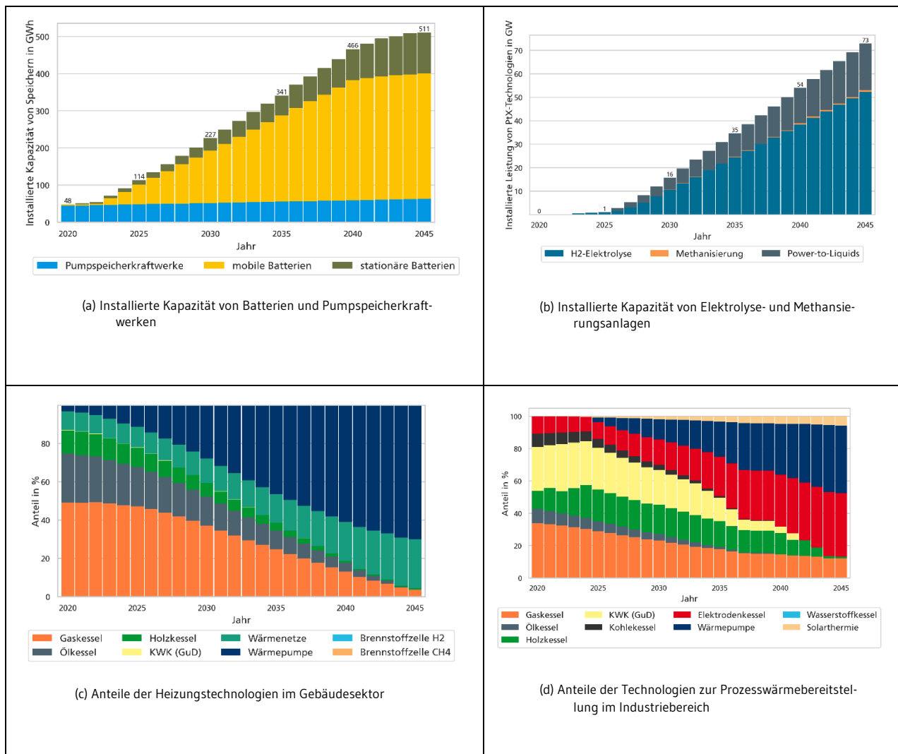
Abbildung 2: Übersicht der wichtigsten Ergebnisse in Bezug auf Leistungen und Anteile in verschiedenen Bereichen des Energiesystems
