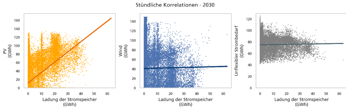
Abbildung 18: Korrelationen Beladen von Energiespeichern im Jahr 2030
