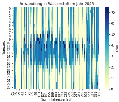
Abbildung 21: Stromverwendung der Elektrolyseure im Jahr 2045
