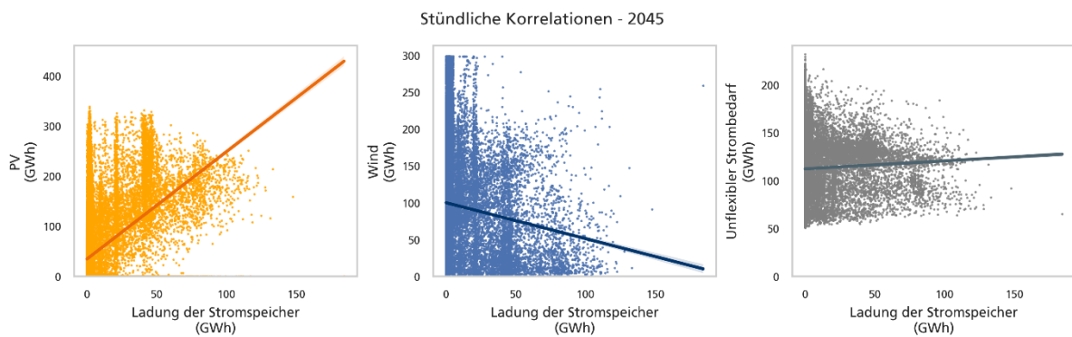
Abbildung 19: Korrelationen Beladen von Energiespeichern im Jahr 2045
