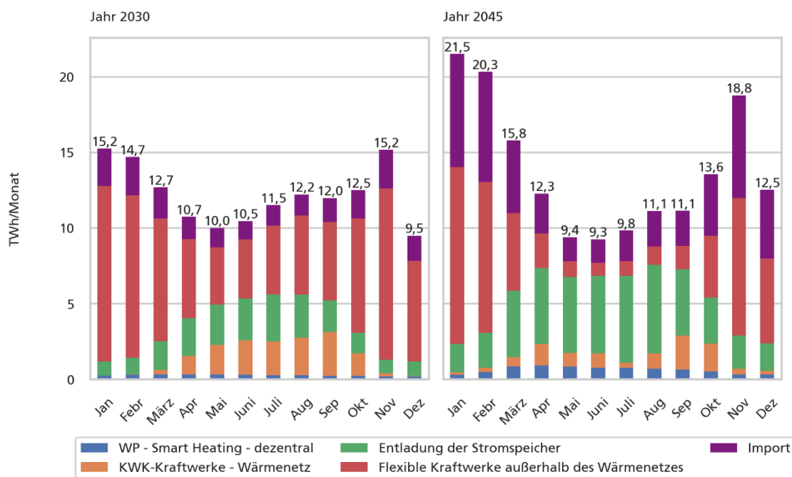
Abbildung 11: Monatlicher Flexibilitätseinsatz bei Strommangel in den Jahren 2030 und 2045. Smart Heating beschreibt hier die Lastverschiebung des Einsatzes von Wärmepumpen und den dadurch in Stunden mit Strommangel eingesparten Strombedarf
