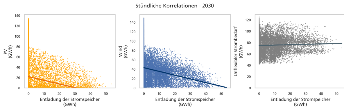
Abbildung 16: Korrelationen der Speicherentladung im Jahr 2030
