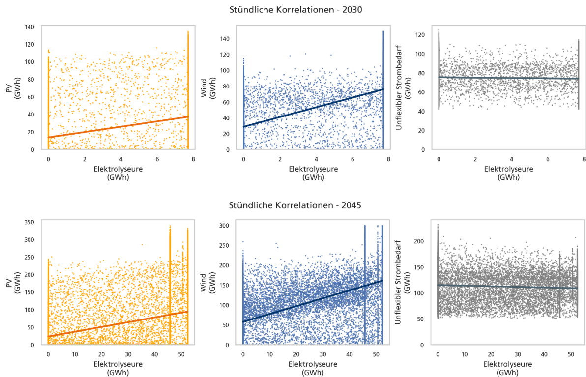
Abbildung 23: Betrieb von Elektrolyseuren auf der x-Achse in Abhängigkeit von Erzeugung aus PV und Wind sowie unflexiblem Bedarf auf der y-Achse für 2030 (oben) und 2045 (unten). Zudem ist jeweils die Regressionsgerade eingezeichnet.
