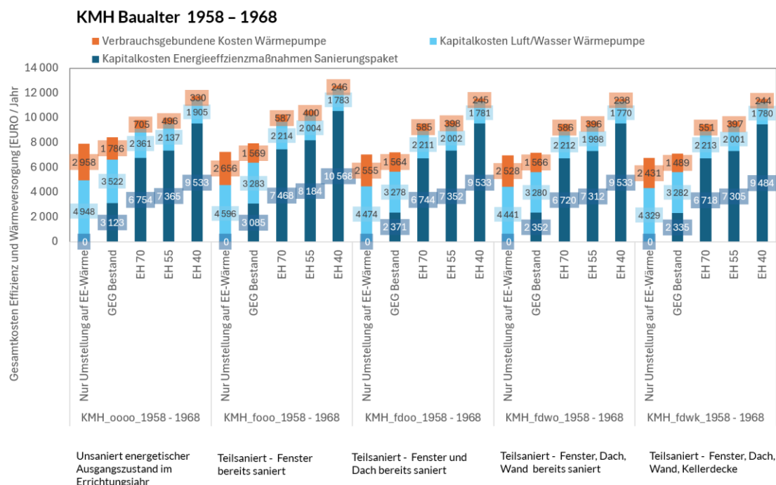
Abbildung 37: Jahresgesamtkosten aus Effizienzmaßnahmen und Wärmeversorgung ausgewählter Referenzgebäudeklassen im Mehrfamilienhäuserbestand
