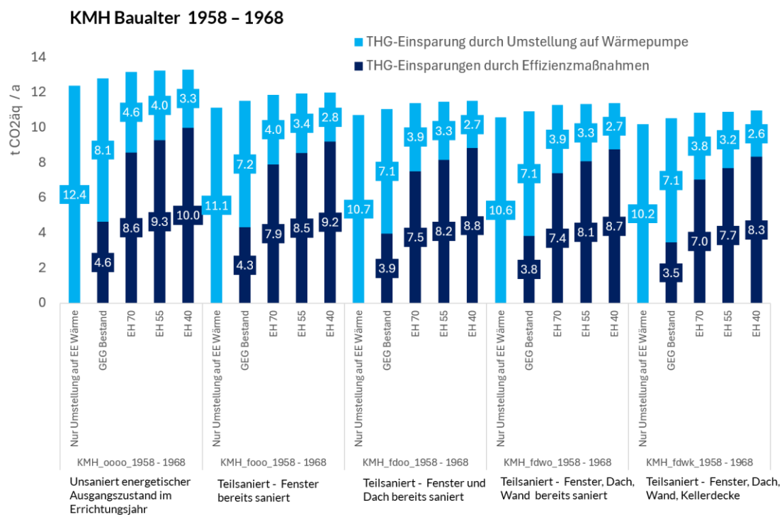
Abbildung 39: Direkte THG-Emissionseinsparungen Referenzgebäudeklasse kleine Mehrfamilienhäuser 1958 – 1968
