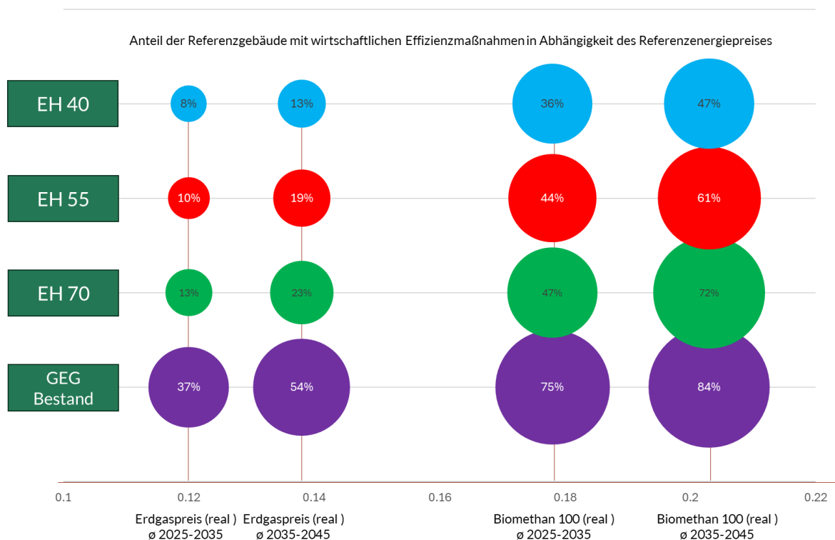
Abbildung 22: Zusammenfassung Anteil wirtschaftlicher Effizienzmaßnahmenpakete bei unterschiedlichen Energiepreisen und einer Abschreibungsdauer von 60 Jahren
