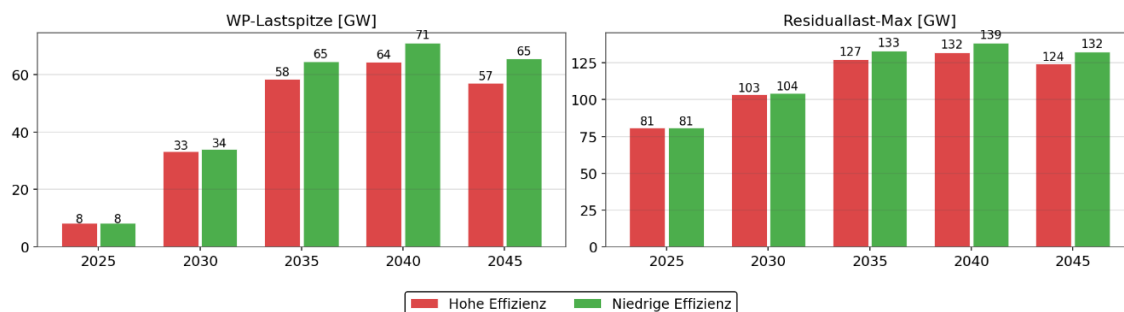
Abbildung 67: Vergleich der Strom-Lastspitzen und maximalen Residuallasten durch Wärmepumpen beider Effizienzscenarien
