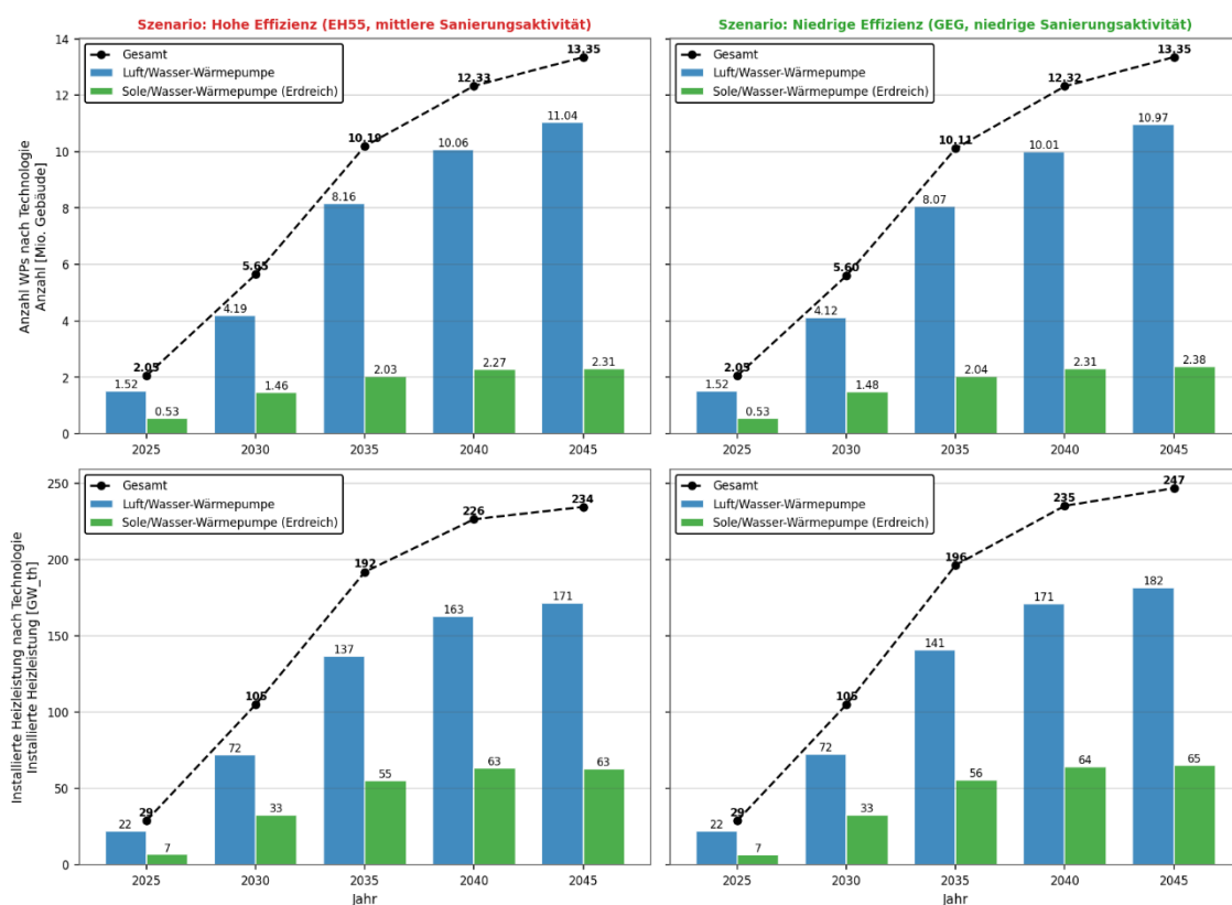
Abbildung 58: Anzahl und thermische Leistung installierter Wärmepumpen in beiden Effizienzsznarien im Simulationszeitraum 2025 bis 2045
