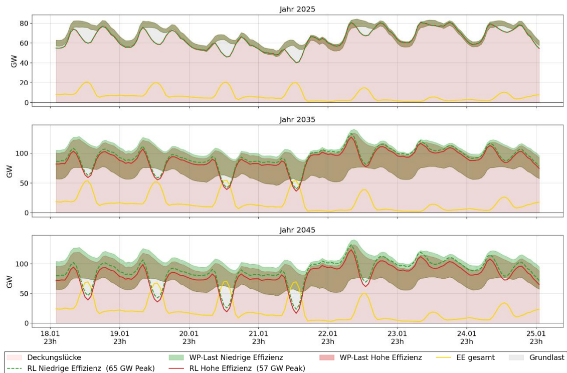
Abbildung 68: Vergleich der WP-Stromlasten zwischen den Effizienzszenarien während einer Dunkelflautewoche
