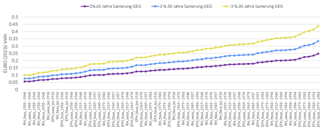
Abbildung 25: Energieeinsparkosten Sensitivitäten: Annuität der Investitionen pro eingesparte Kilowattstunde Nutzwärme [EURO/kWh] – Einfamilienhäuser und Reihenhäuser
