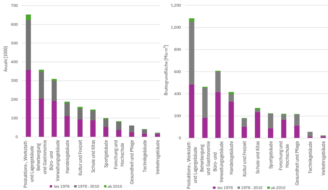
Abbildung 8: Bruttogrundfläche und Anzahl nach Gebäudetyp und Baualtersklasse im Nichtwohngebäudebestand
