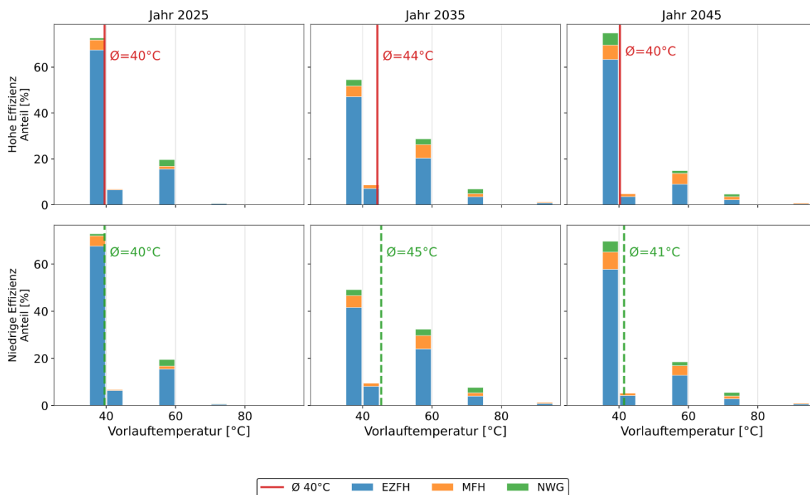
Abbildung 74: Relative Verteilung an Gebäuden mit Wärmepumpe nach Vorlauftemperatur für das Hoch- und NiedrigeffizienzszENARIO
