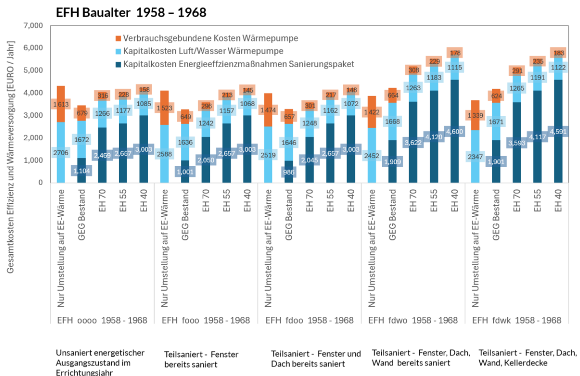
Abbildung 36: Jahresgesamtkosten aus Effizienzmaßnahmen und Wärmeversorgung ausgewählter Referenzgebäudeklassen im Einfamilienhausbestand
