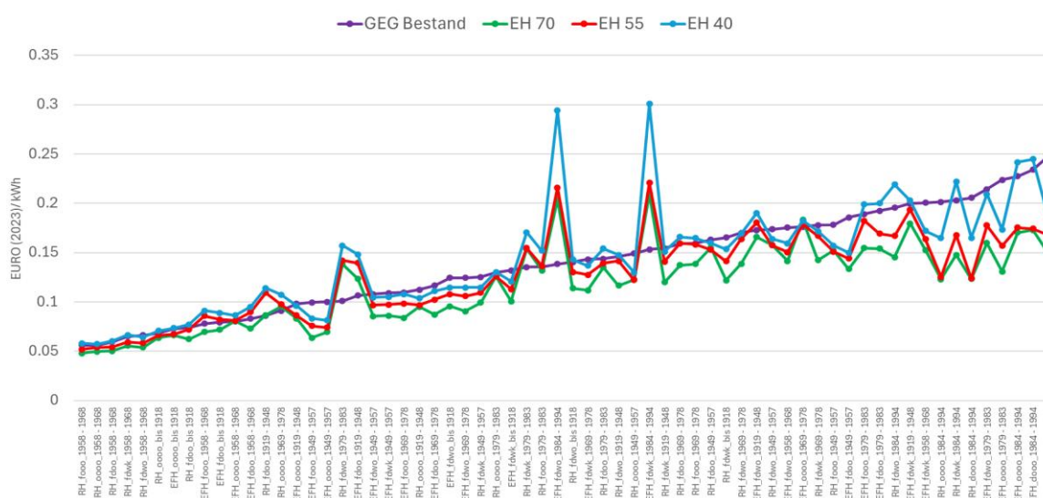
Abbildung 23: Energieeinsparkosten: Annuität der Investitionen pro eingesparte Kilowattstunde Nutzwärme [EURO/kWh] – Einfamilienhäuser und Reihenhäuser (inkl. Förderung)
