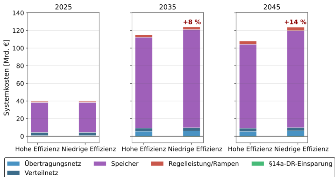
Abbildung 72: Vergleich der geschätzten jährlichen Kosten aufseiten des Stromsystems durch unterschiedliche Wärmepumpen-Stromlasten zwischen beiden Effizienzszenarios
