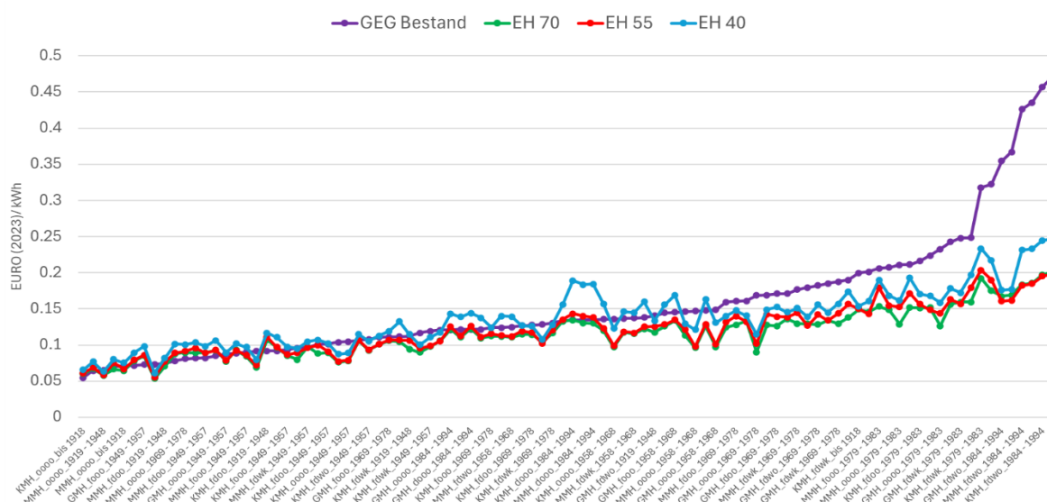
Abbildung 24: Energieeinsparkosten: Annuität der Investitionen pro eingesparte Kilowattstunde Nutzwärme [EURO/kWh] – Mehrfamilienhäuser (inkl. Förderung)
