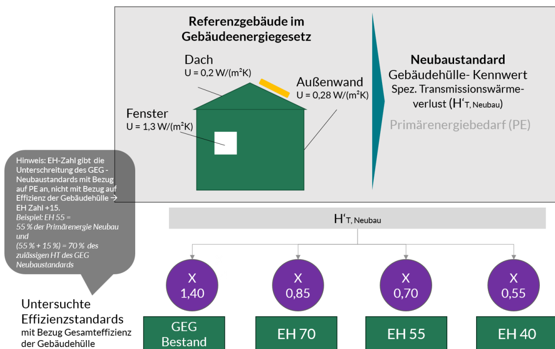
Abbildung 5: Untersuchte Effizienzstandards mit Bezug auf die Mindesteffizienz der Gebäudehülle
