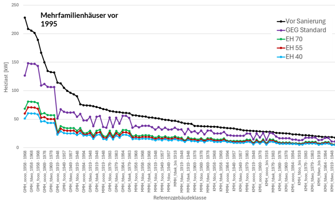
Abbildung 32: Heizlast eines Mehrfamilienhaus-Referenzgebäudes vor und nach Sanierung
