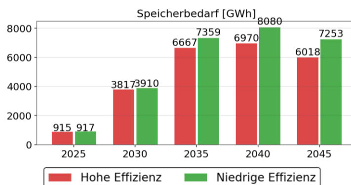
Abbildung 70: Vergleich des Speicherbedarfs in beiden Effizienzszenarios bei Annahme eines vollständigen Ausgleichs der Residuallast durch saisonale Speicher
