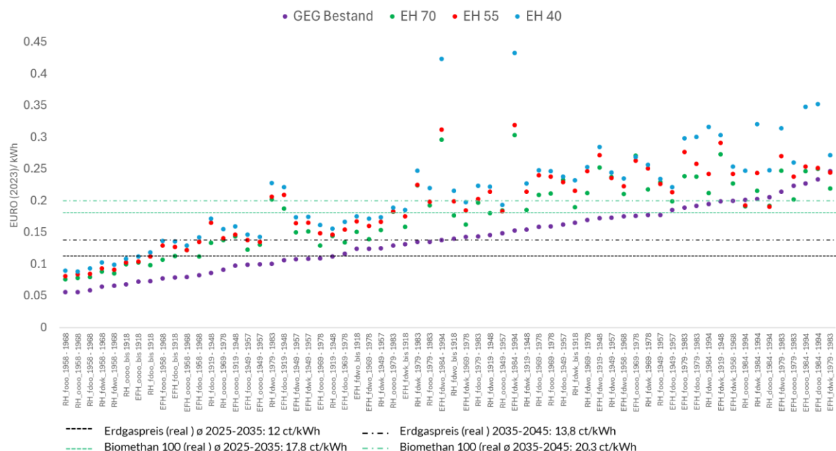
Abbildung 20: Energieeinsparkosten: Annuität der Investitionen pro eingesparte Kilowattstunden Nutzwärme [EURO/kWh] bei einer Abschreibungsdauer von 60 Jahren – Einfamilienhäuser und Reihenhäuser (ohne Förderung)
